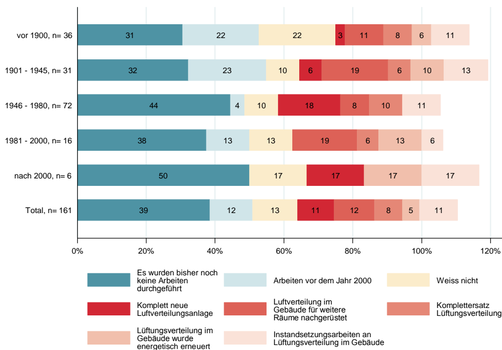
Figur 32: Durchgeführte Arbeiten an Luftverteilung. Antworten auf die Frage: «Bitte geben Sie an, welche Arbeiten zwischen 2000 und 2012 an der Luftverteilung/-abgabe durchgeführt wurden.»
