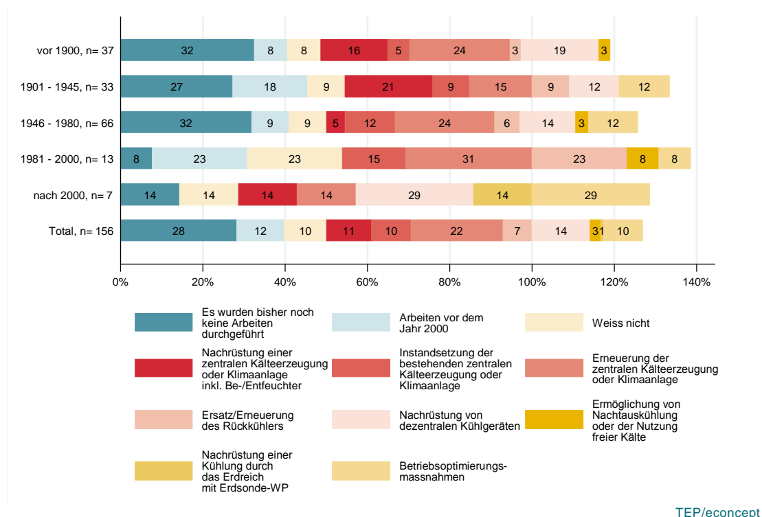
Figur 31: Durchgeführte Arbeiten an Kälteerzeugung. Antworten auf die Frage: «Bitte geben Sie an, welche Arbeiten zwischen 2000 und 2012 an der Kälteerzeugung durchgeführt wurden.»
