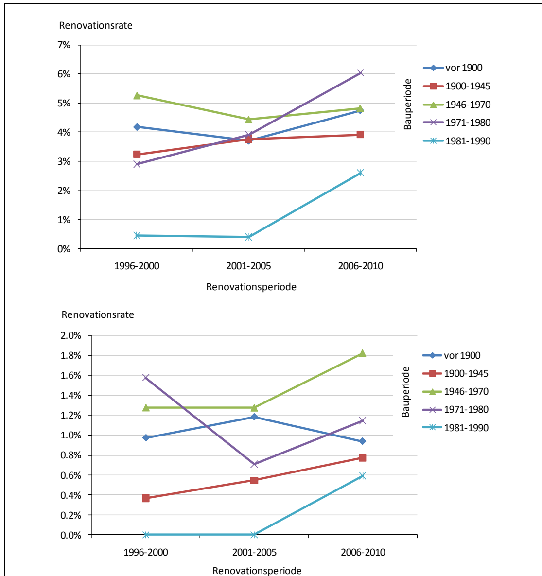
Figur 6: Zeitlicher Verlauf der jährlichen Renovationsrate energieeffizienter Massnahmen am Beispiel der Gebäudeelemente Fenster (oben) und Fassade (unten). (Rate relativ zur Anzahl Gebäude beim jeweiligen Gebäudeelement, welche vor der entsprechenden Renovationsperiode in den Besitz des Eigentümers gelangt sind)
