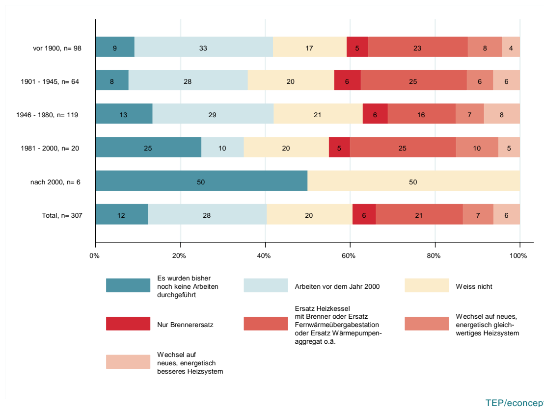
Figur 27: Durchgeführte Arbeiten an Heizung. Antworten auf die Frage: «Bitte geben Sie an, welche Arbeiten zwischen 2000 und 2012 an der Heizung durchgeführt wurden.»
